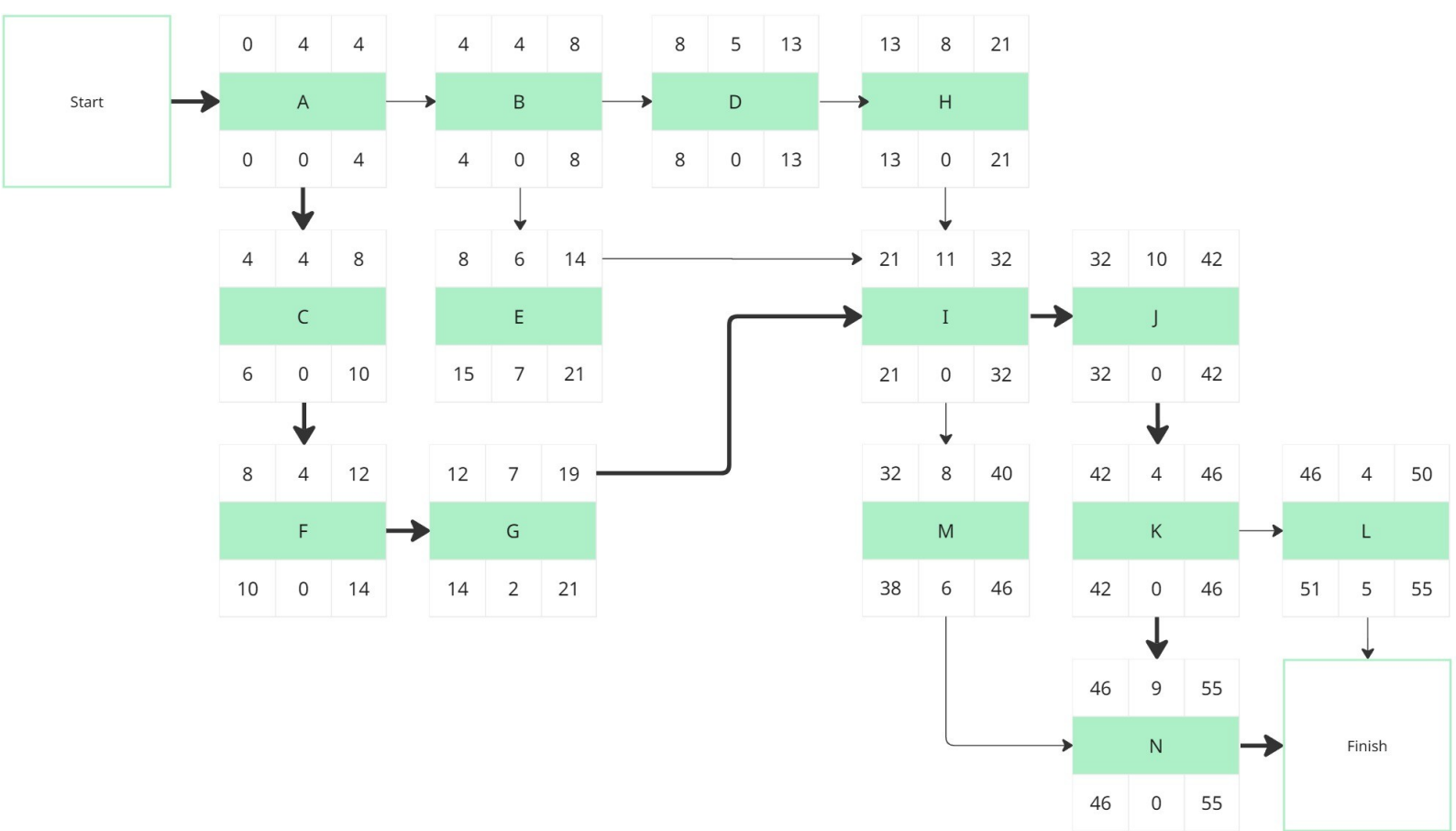
Рисунок 2.2 — Діаграма передування з критичним шляхом
